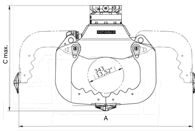
optionale 4-Grip Ansteckvorrichtung, hier angebaut an einem A06HPX
